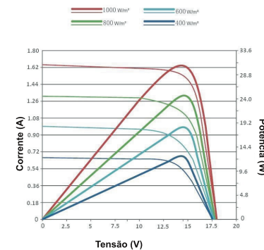
Curvas Corrente-Tensão & Potência-Tensão
